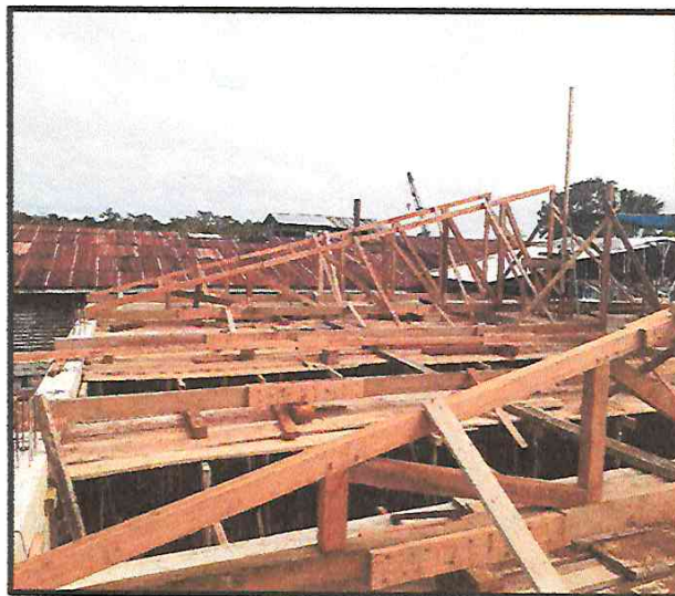
INSTALACIÓN DE TIJERALES DE MADERA.
