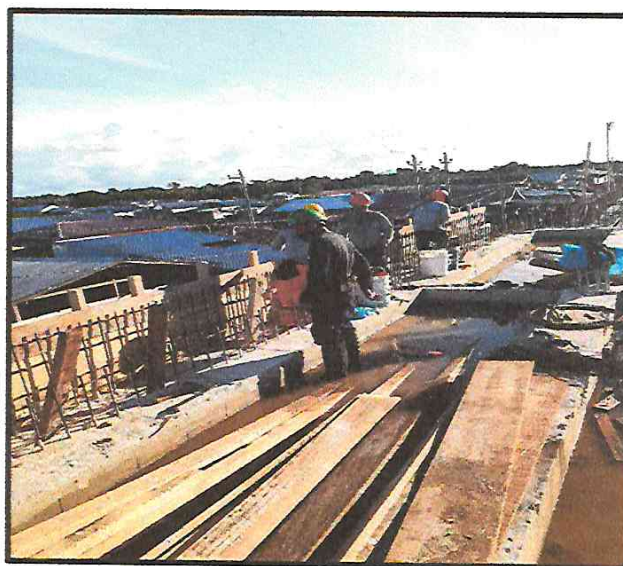
ENCOFRADO DE PARAPETOS.
