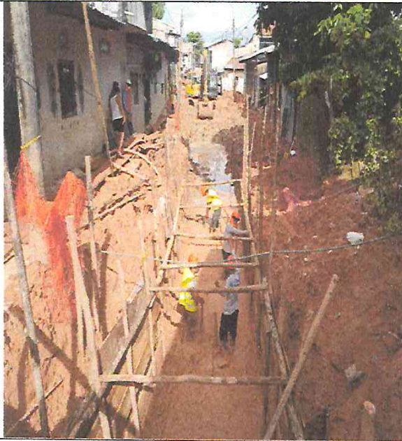
Excavación de zanja y entibado de paredes en calle prolongación Jose Galvez.
