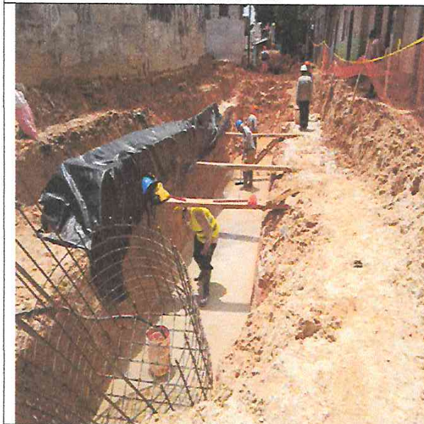
Colocación de acero corrugado en alcantarillas y buzones.
