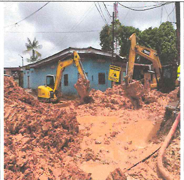
Suelo saturado a causa de precipitaciones pluviales.
