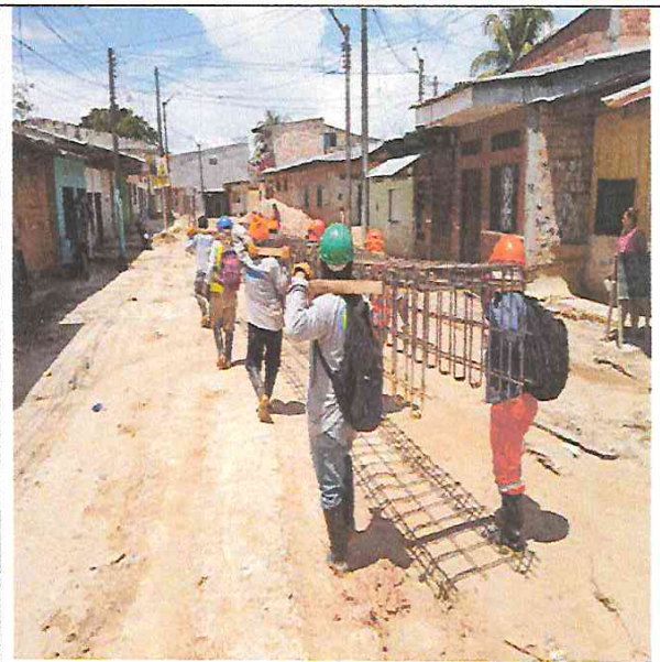
Colocación de acero corrugado en alcantarillas.
