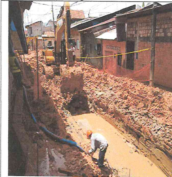
Excavación de zanja canal en calle prolongación Jose Gálvez.
