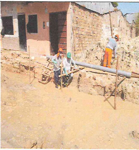
Colocación e instalación de drenaje auxiliar con tubería de PVC 6" en calle Triangulo de Bermuda.
