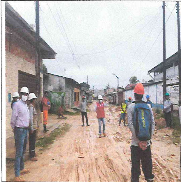
Charla de seguridad y salud en el trabajo.
