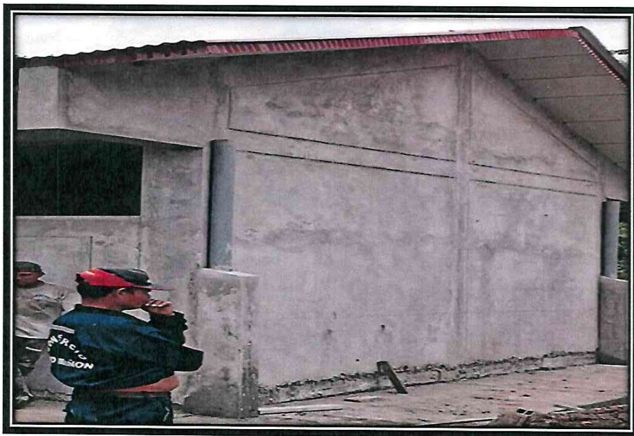
8.00 EN LA FOTO SE PUEDE APRECIAR LA CONSTRUCCION DE MURO PROTECTOR PARA TUBO DE BAJADA DE DRENAJE PLUVIAL h= 1.50 \text{ mts.} Y COLOCACION DE TUBERIA DE BAJADA DE AGUA DE LLUVIA PVC SAL \varnothing 4'' (Inc. Codos PVC SAL), EN LOS DIFERENTES MODULOS.
