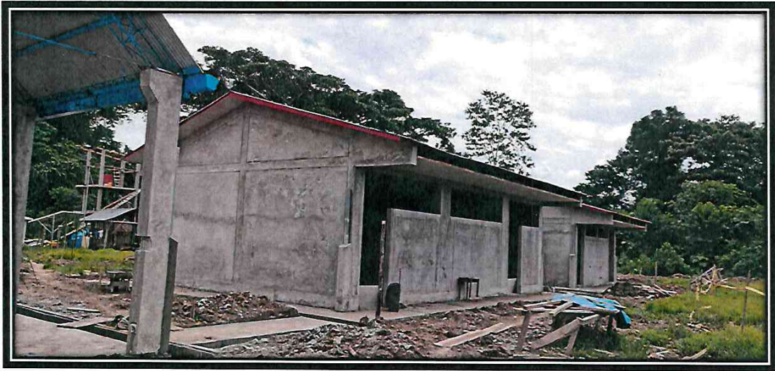
7.00 EN LA FOTO SE PUEDE APRECIAR LA CONSTRUCCION DE VEREDA DE ACCESOS DE MORTERO f'c= 175 \text{ kg/cm}^2 FROTACHADO DE e= 4''
