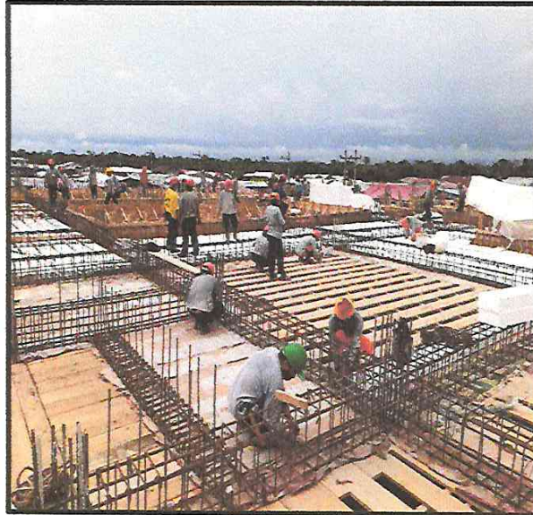
COLOCACIÓN DE MALLA METÁLICA.
