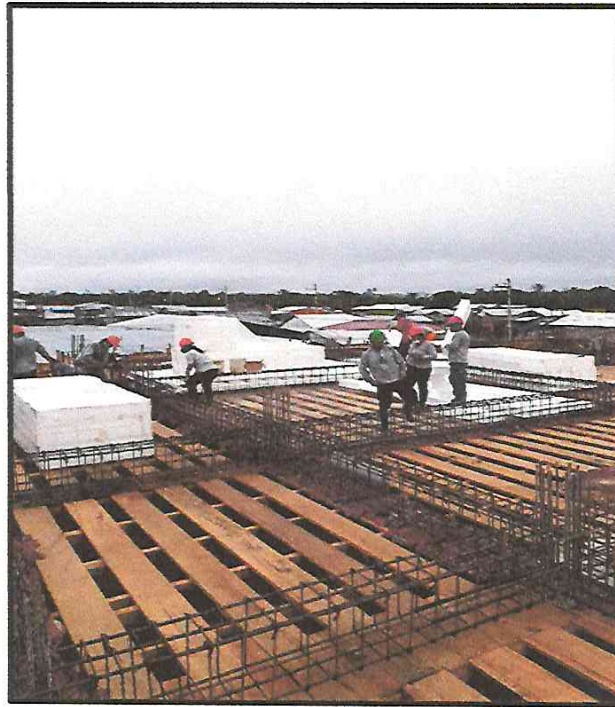
HABILITACIÓN DE TECNOPORT.
