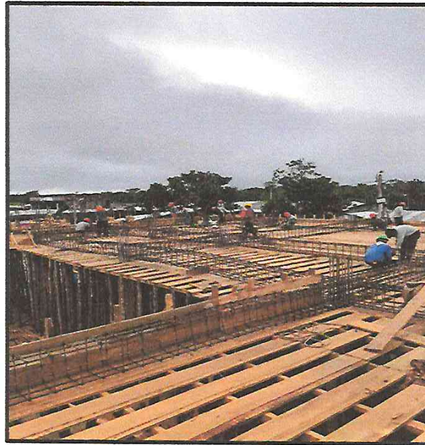
INSTALACIÓN DE ACERO CORRUGADO EN VIGAS.
