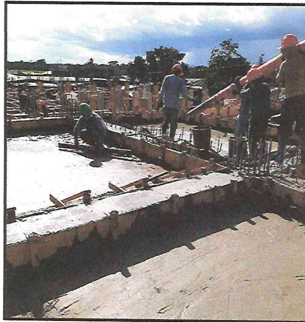
VACEO DE LOSA ALIGERADA.
