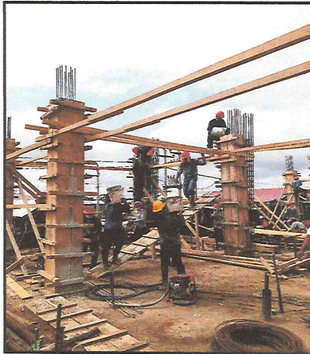
VACEO EN COLUMNAS.
