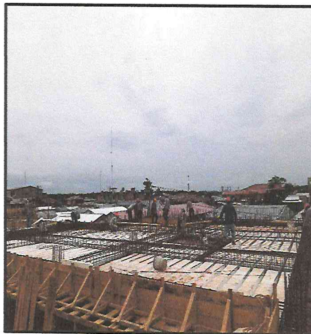
HABILITACIÓN E INSTALACIÓN DE BLOQUES DE TECNOPORT.
