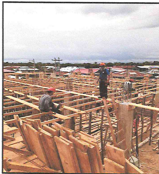
ENCOFRADO PARA LOSA ALIGERADA.
