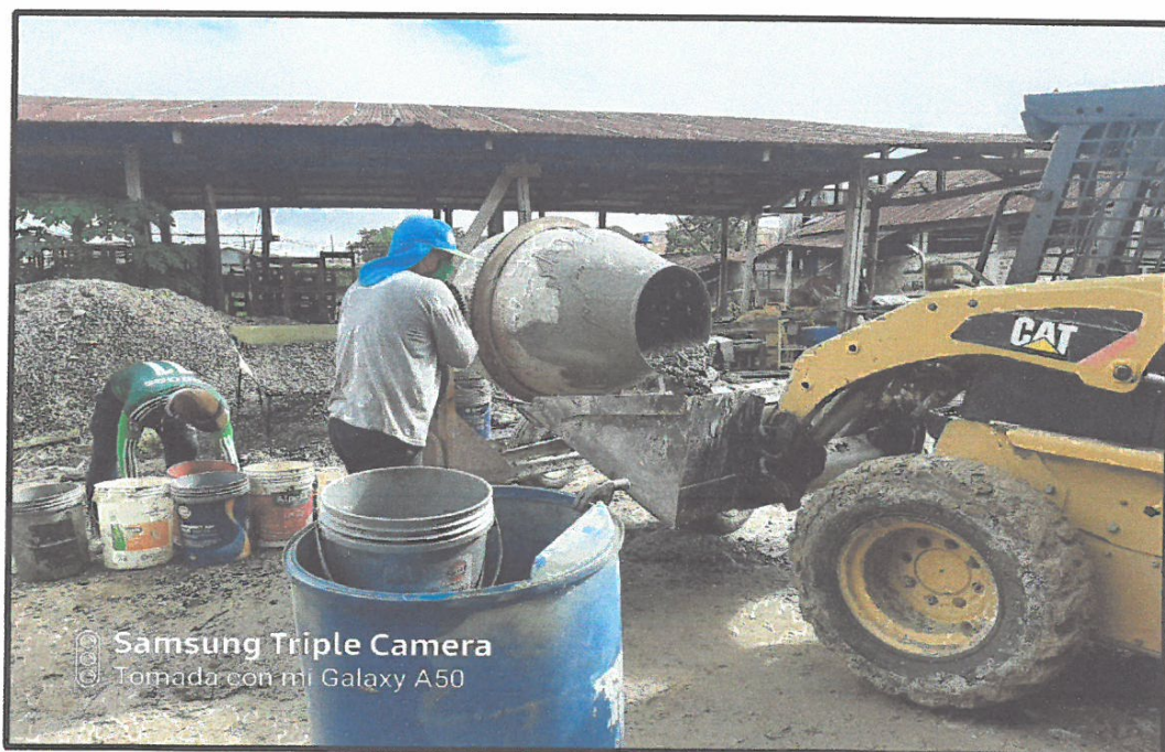
VACIADO DE CONCRETO ARMADO F'C=280KG/CM2 PARA PILOTES DE 0.50 X 0.50.
