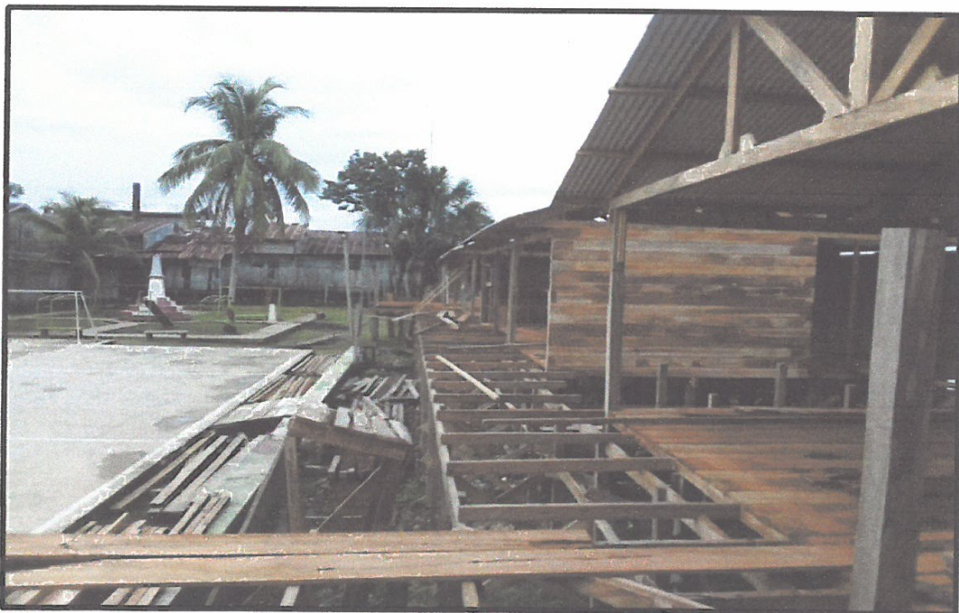
EN LA VISTA PODEMOS APRECIAR LOS TRABAJOS DE OBRAS PROVISIONALES (OFICINAS ADMINISTRATIVAS, COMEDOR, ALMACEN, GARITA DE VIGILANCIA, SS.HH) REALIZADOS EN OBRA.
