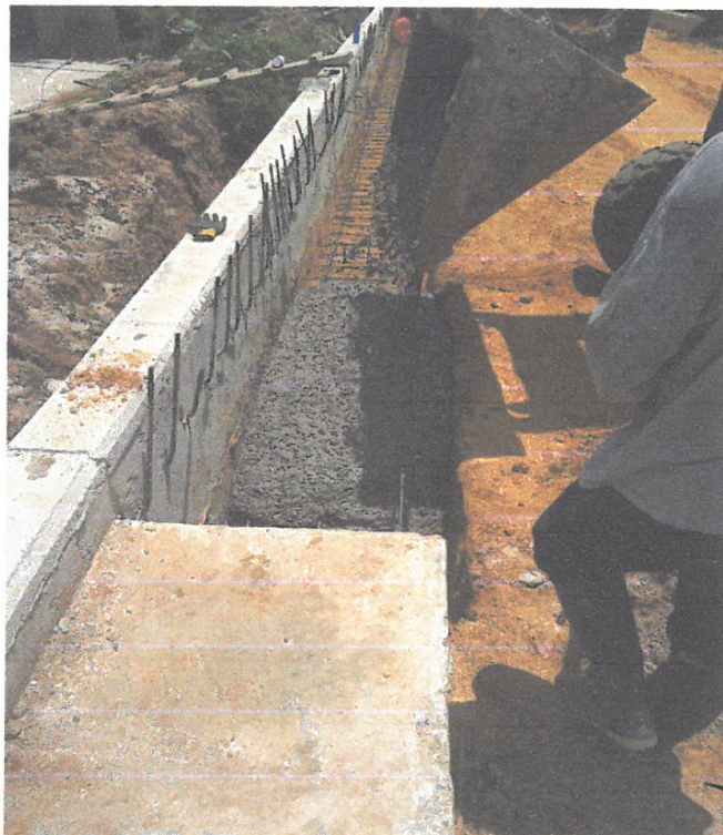
VACEO DE PISO DE CUNETETA EN LA CALLE CONDAMINE CUADRA 03-LADO DERECHO.
