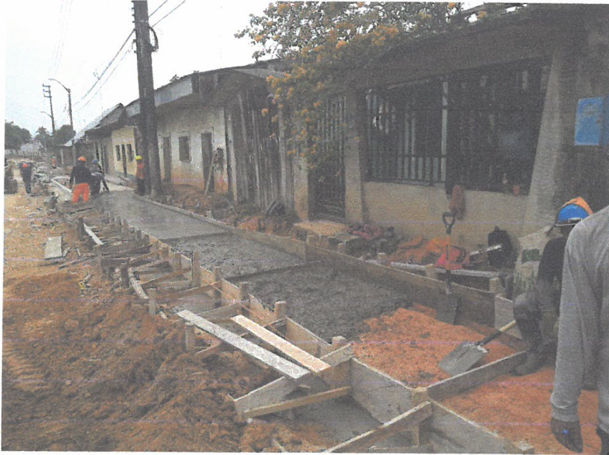
VACEO DE VEREDA EN LA CALLE RAYMONDI CUADRA 01, LADO IZQUIERDO.
