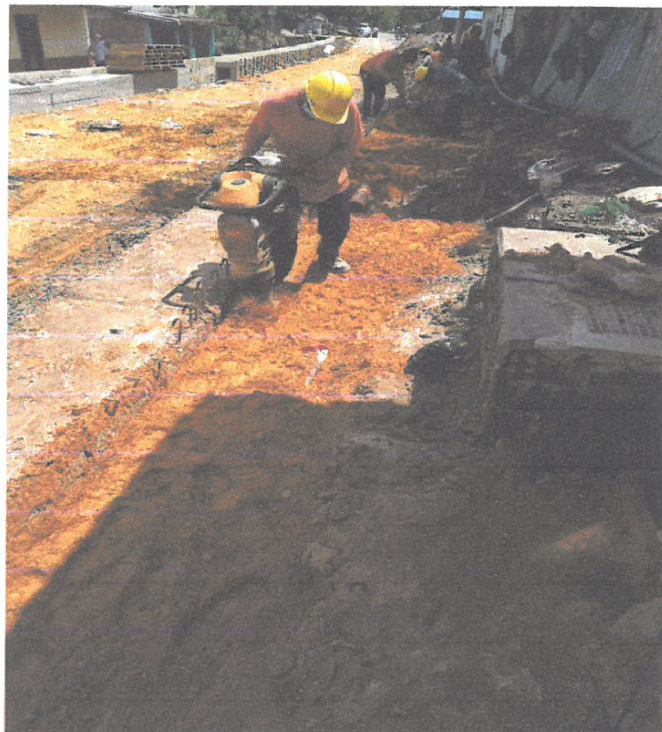
COMPACTACION DE MATERIAL MEJORADO PARA ENCOFRADO DE VEREDA EN LA CALLE CONDOMINE CUADRA 03-LADO IZQUIERDO.
