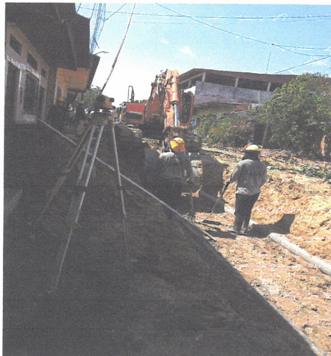
EXCAVACION DE ZANJA PARA CUNETA EN LA CALLE MARAÑON CUADRA 04-LADO DERECHO.
