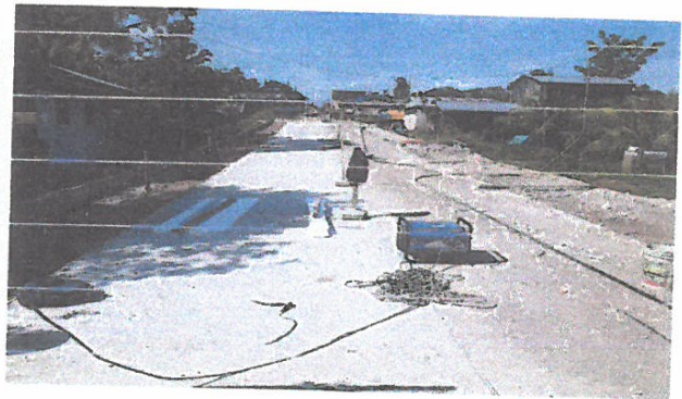
TERMINADO DE CONCRETO F'C=210 KG/CM2, EN JR. 2 DE MAYO, ENTRE JR. ALFONSO UGARTE Y JR. SAN MARTIN
