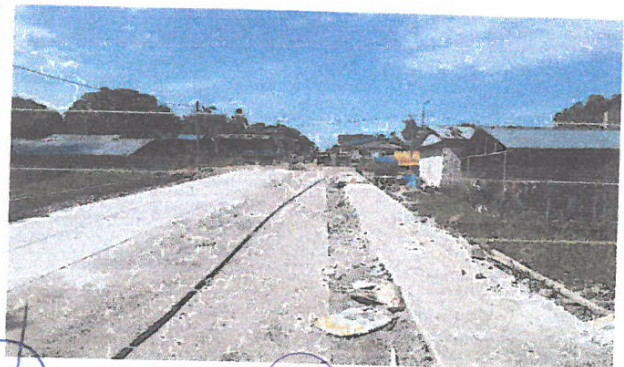
VEREDAS VACIADAS Y PULIDAS CON CONCRETO F'C=175 KG/CM2, EN JR. 2 DE MAYO, ENTRE JR. ALFONSO UGARTE Y JR. SAN MARTIN
