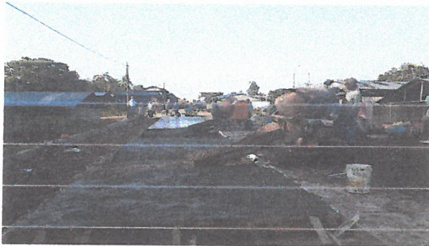
VACIADO DE CONCRETO F'C=210 KG/CM2, EN JR. 2 DE MAYO, ENTRE JR. ALFONSO UGARTE Y JR. SAN MARTIN
