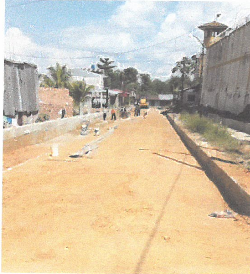
MEJORAMIENTO Y COMPACTACION, PARA ENCOFRADO DE PISO DE CUNETA EN LA CALLE TARATA CUADRA 07, LADO DERECHO.
